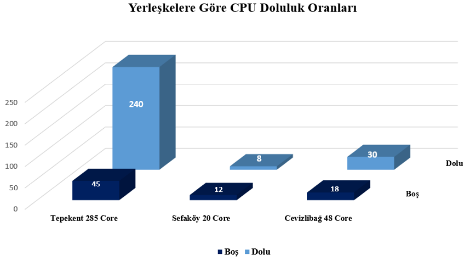
Şekil IX.5.CPU Doluluk Durumu
